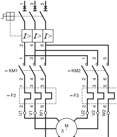
有成套保护 GV2LE
