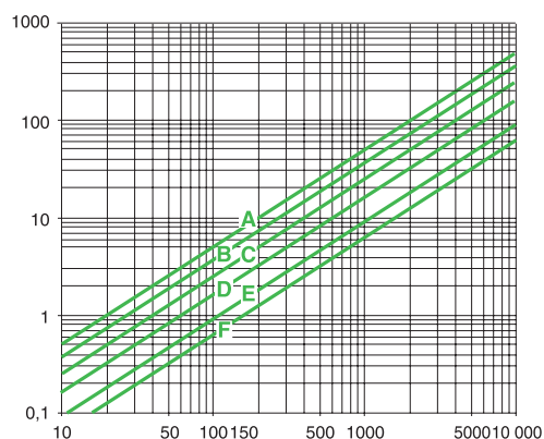
控制回路中两根导线的总阻值 (1)
