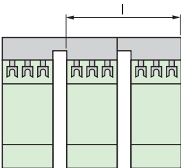
母排 GV2G345 和 G354
