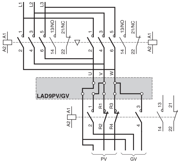
低速 / 高速配线组件、螺钉夹紧端子
