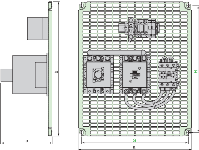
3 x LC1D115 或 D150 或 D170
