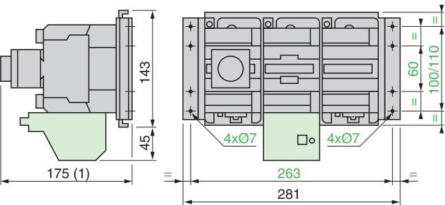
3 x LC1D40A 或 D50A
