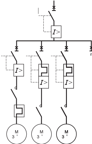
有成套保护 GV2LE
