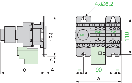
3 x LC1D09 到 D32
