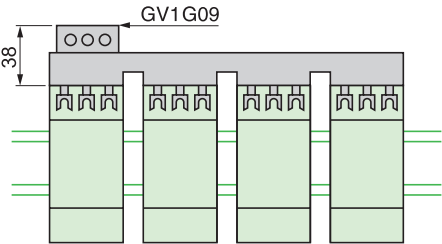
母排 GV2G●●● 带接线端子模块 GV1G09
