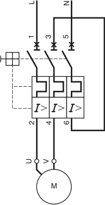
单相或直流电动机 GV2ME , GV2PM
